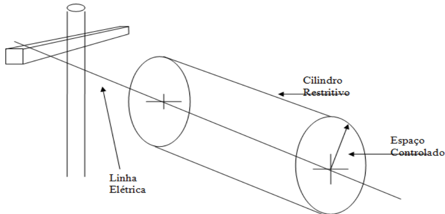
Figura 03 – Cilindro restritivo para operação de equipamento de levantamento
